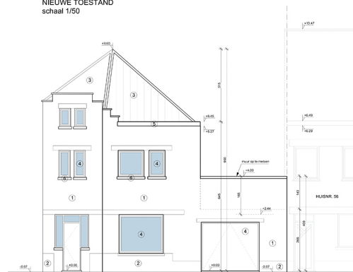
VOORGEVEL NIEUWSTRAAT
