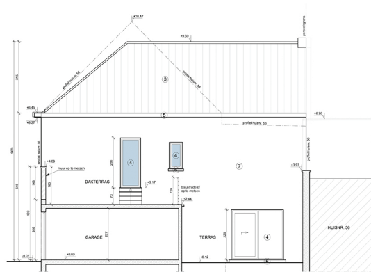
DOORSNED E A-A / ACHTERGEVEL
